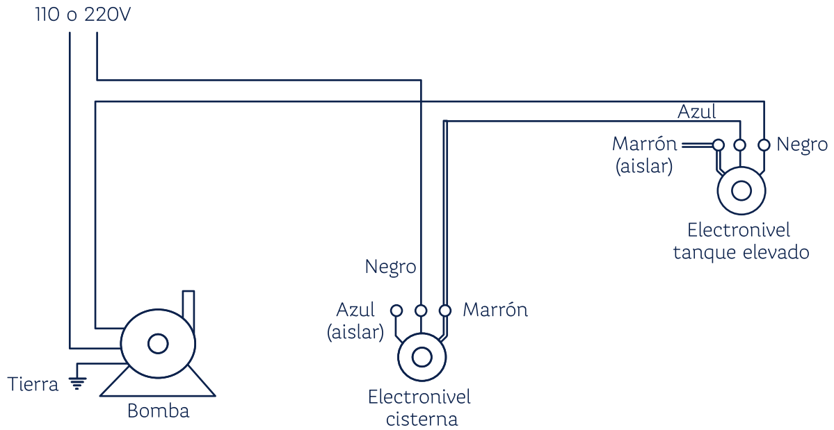
Diagrama Eléctrico
